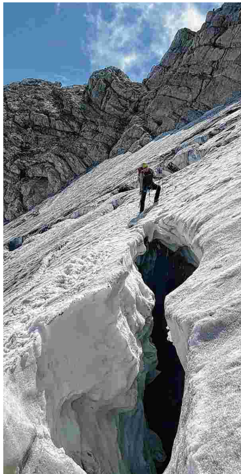
Riesige Gletscherspalten haben sich auf dem Dachstein aufgetan. Foto: Hans Prugger
